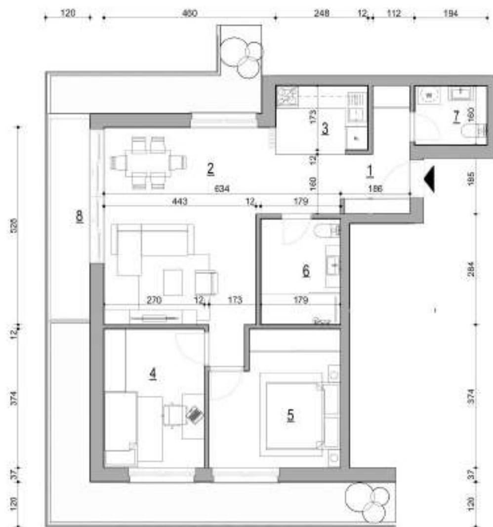
Osnova stana A2-4.10
