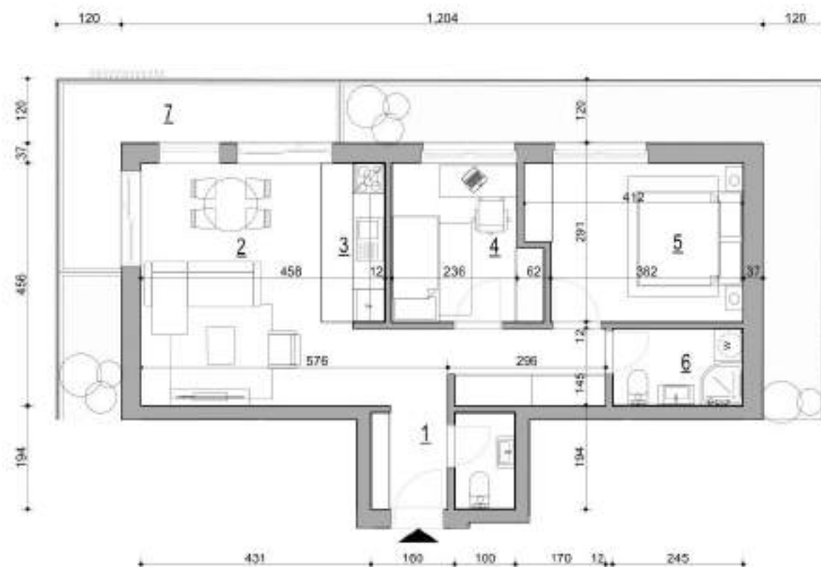
Osnova stana A1-4.05
