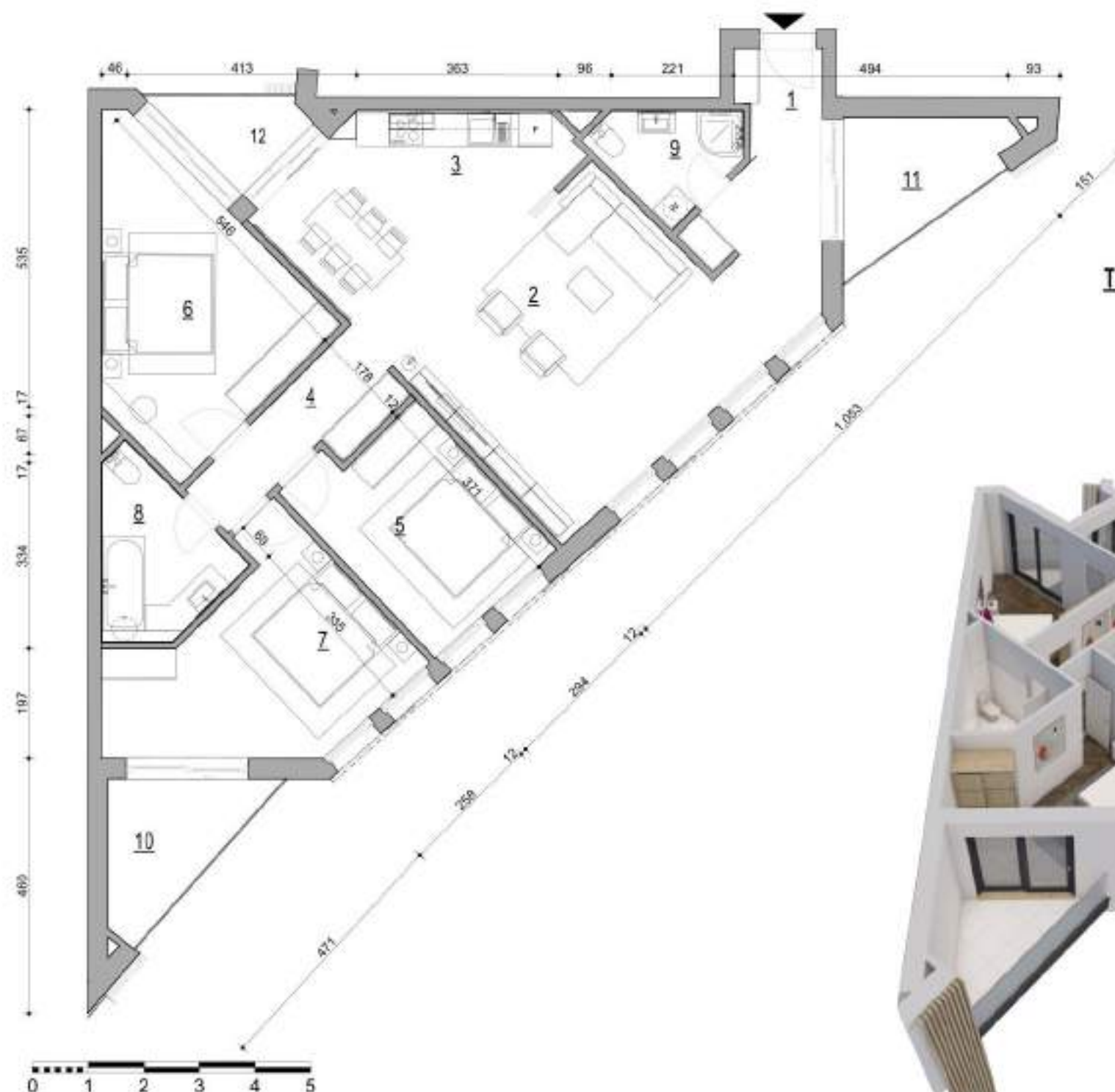
Osnova stana A4-1.08
