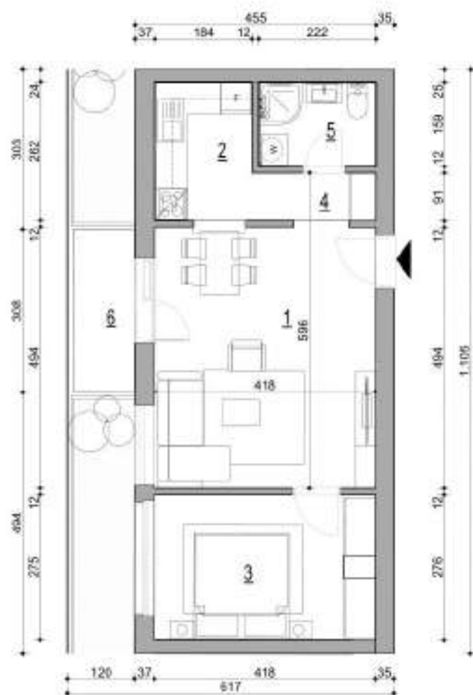
Osnova stana A3-4.10
