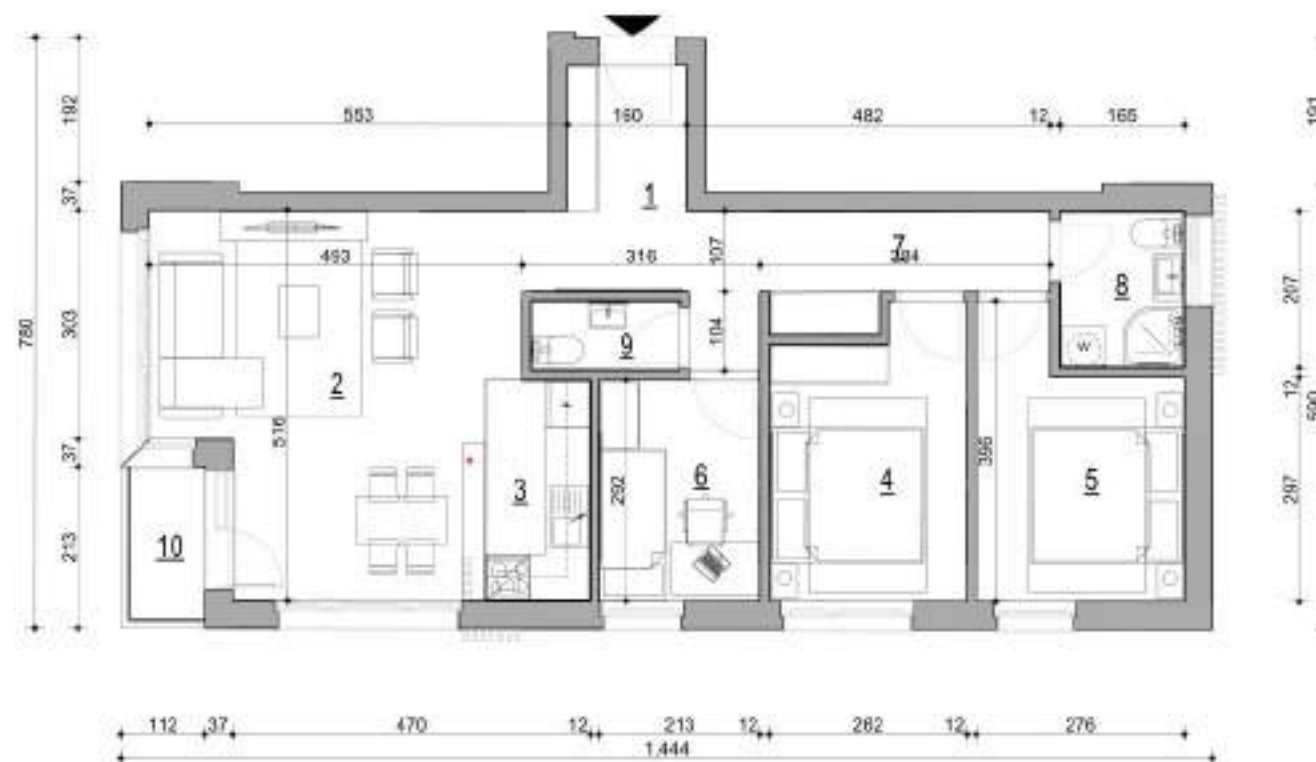
Osnova stana A1-0.06
