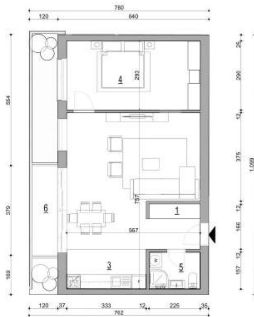
Osnova stana A2-4.11
