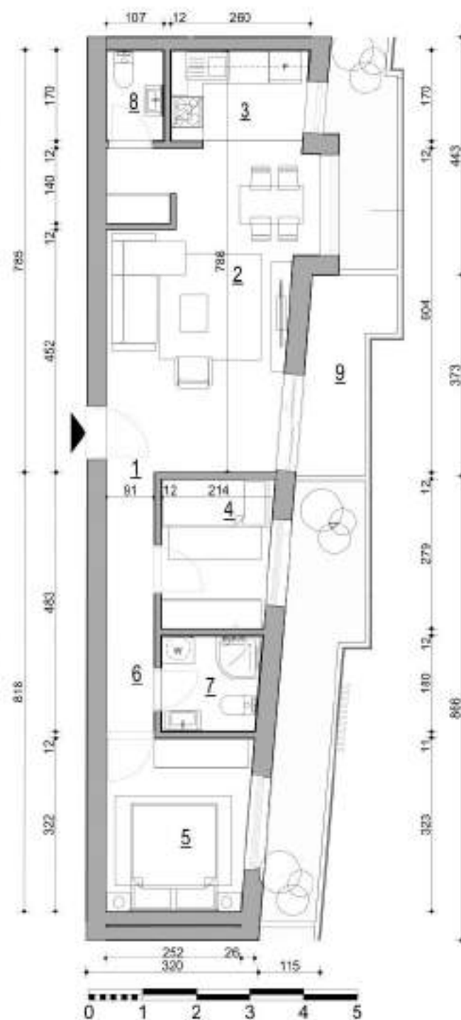
Osnova stana A4-4.08
